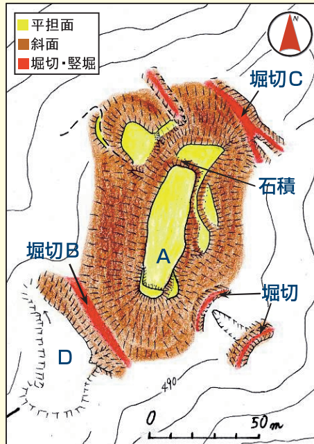
桜尾城略測図(作図 秋本哲治)
