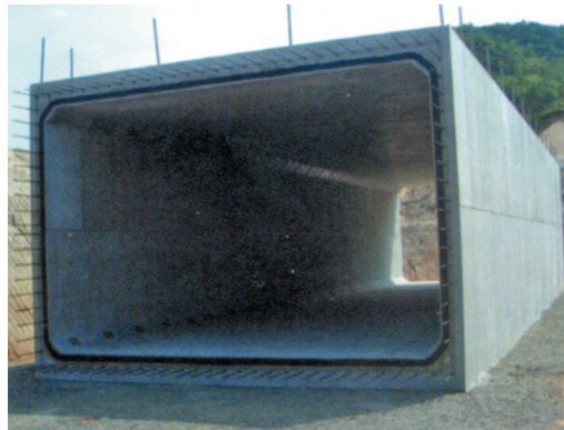
■ボックスカルバート写真 水路・通路・道路などに利用されるプレキャストボックスカルバート。現場作業の省力化・品質の向上を図ります。
