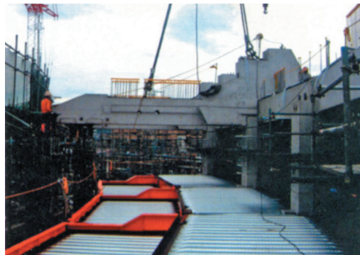
■新市民球場(3塁側2階席)写真 複雑な形状で、高い精度が必要なプレキャストプレストレス構造。柔軟な対応で、高い技術が支えています。
